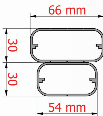
Braccio Serie 300
