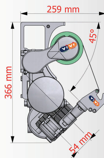
Vista Tenda 45°:
