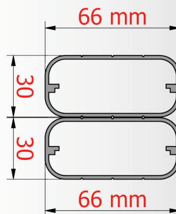
Braccio Serie 350
